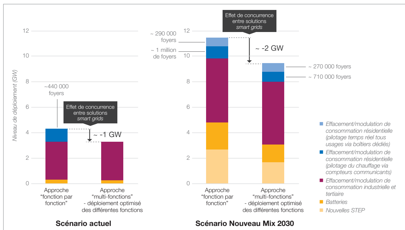
Niveaux de déploiement économiquement pertinents des différentes solutions de flexibilité smart grids
